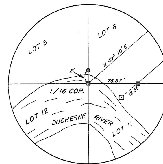
DETAIL N.T.S.
